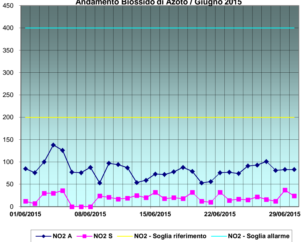
Andamento Biossido di Azoto / Giugno 2015
