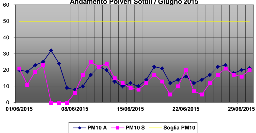
Andamento Polveri Sottili / Giugno 2015
